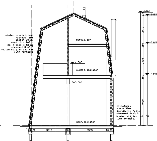
↑ dwarsdoorsnede achter
