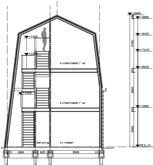
↑ dwarsdoorsnede voor
